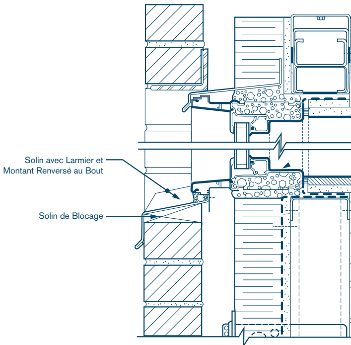
Fig. B Détail d'une Allège de Fenêtre
