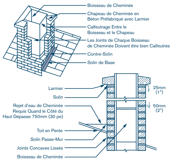
Fig. A Détails d'un Chapeau de Cheminée
