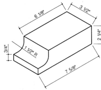
203-Cove Header
